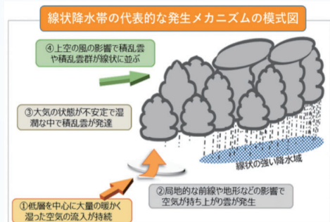
線状降水帯発生メカニズムの模式図
