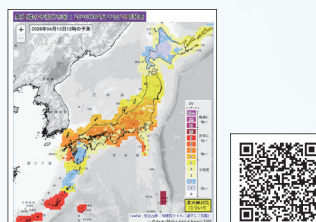
図2 紫外線の予測分布図
