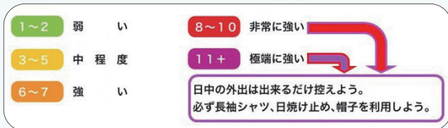
図1 UVインデックス
