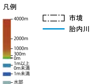
図 1-3 地形の状況
