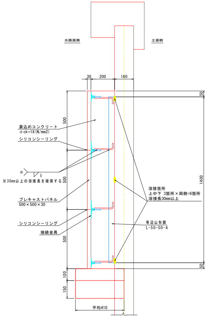
側面図 S=1:10
