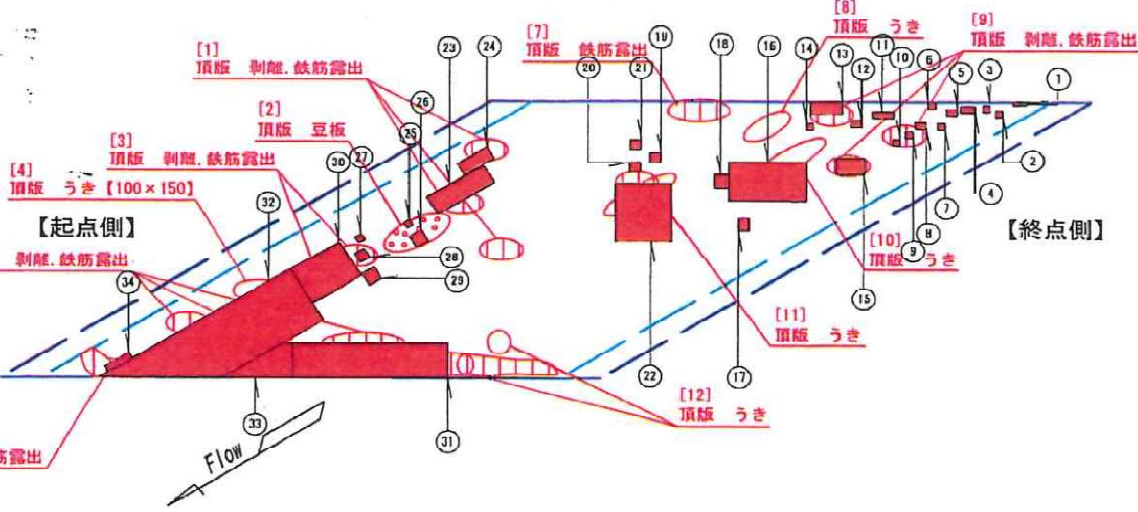
平面図 (頂版)
