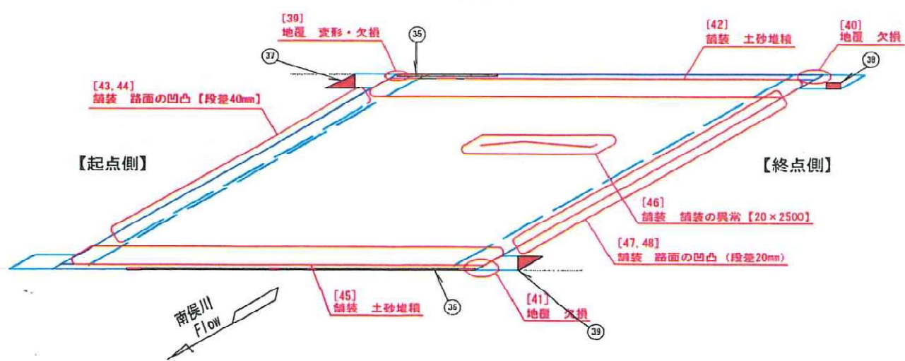
平面図 (橋面)
