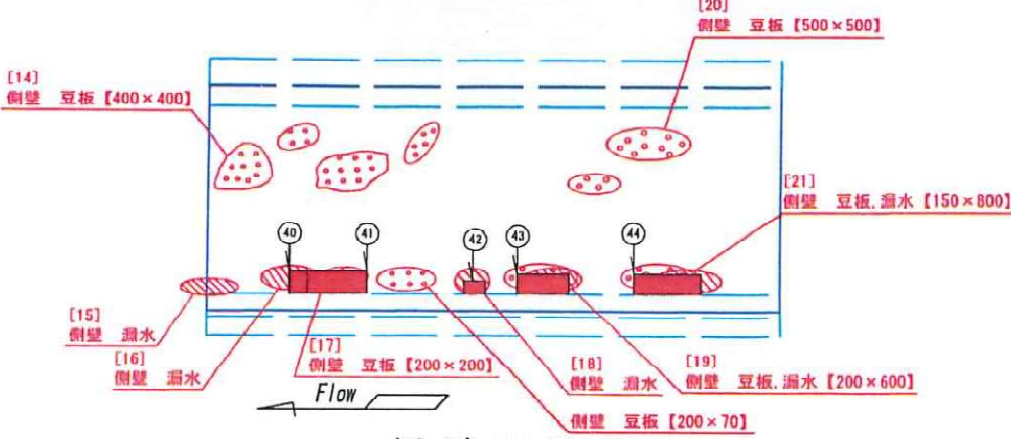
側壁正面図 (終点側)
