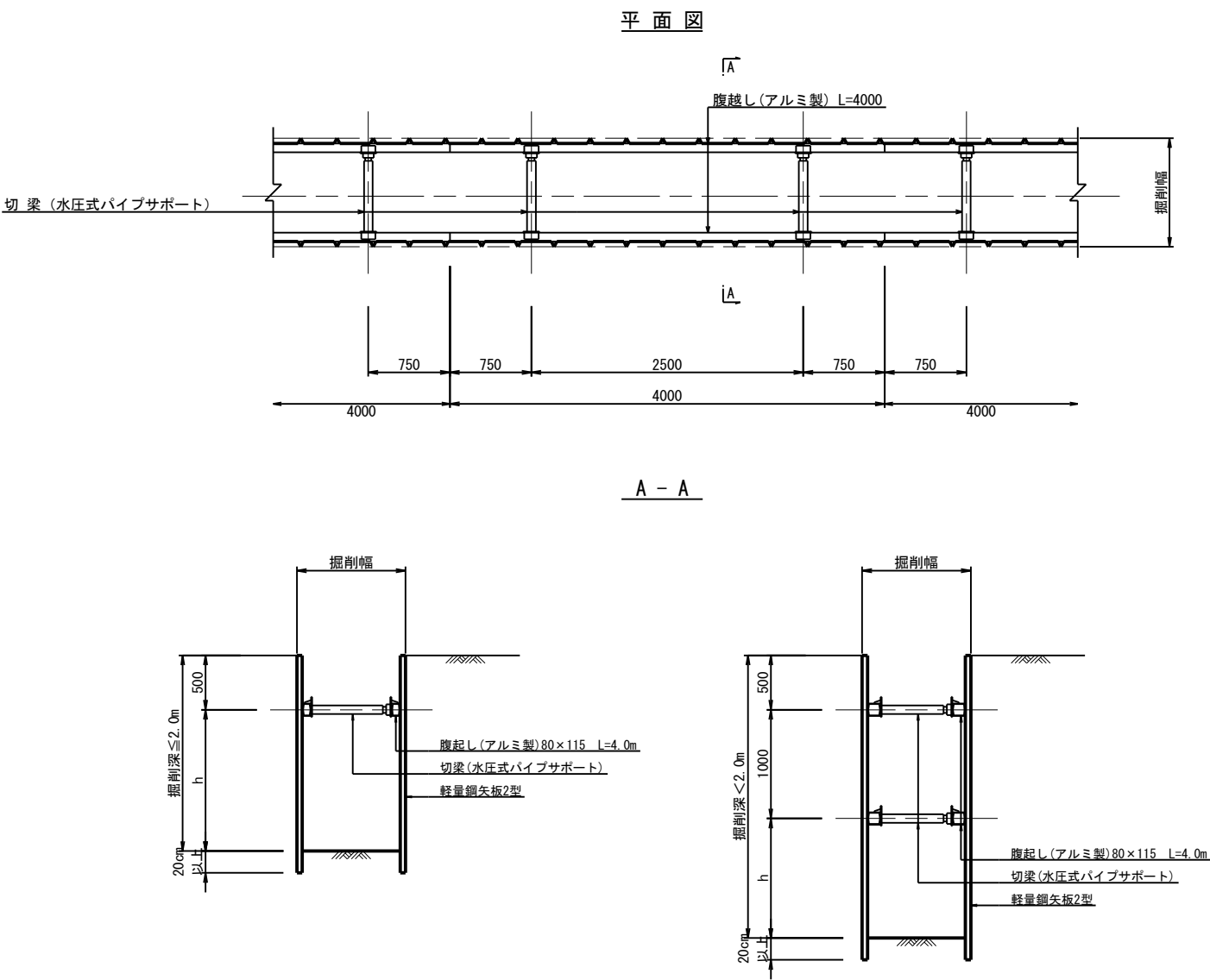
軽量鋼矢板建込工法
