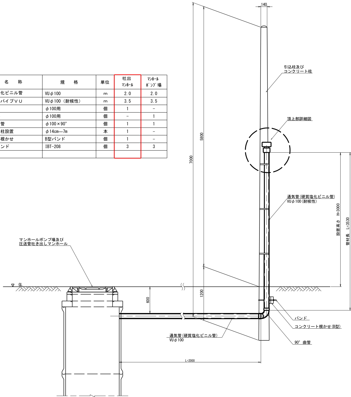
側 面 図
