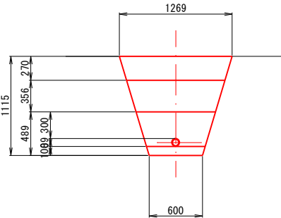
土工図（上流） L=2.5m
