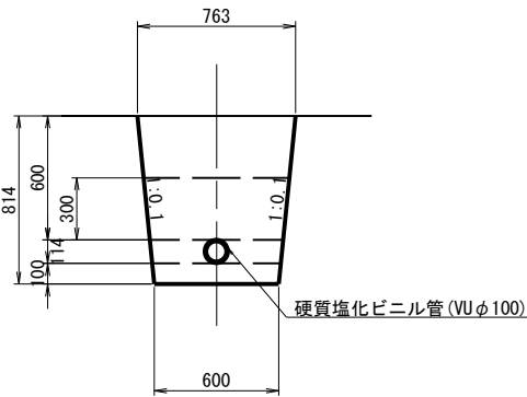
埋設部標準断面 S=1:20
