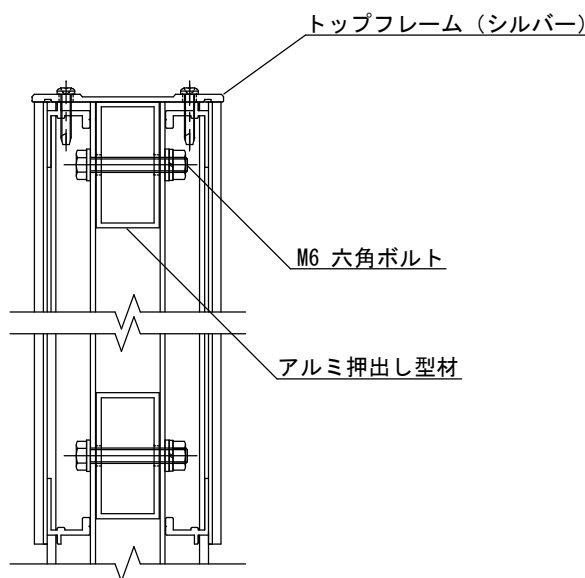
B-B断面詳細図 S=1/3
