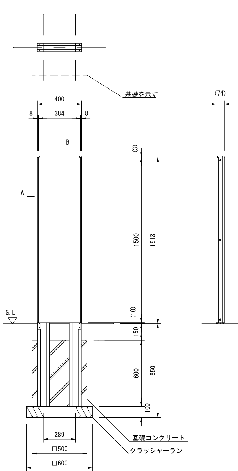
外観図 S=1/20
