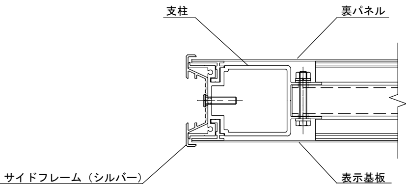
A-A断面詳細図 S=1/3
