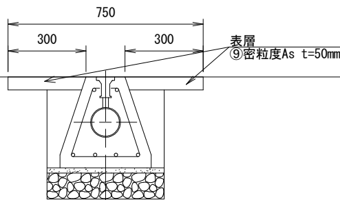
二次施工標準断面図
