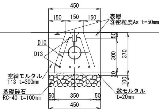
一次施工標準断面図
