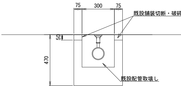
現況断面図
