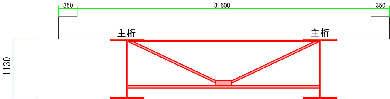
塗替塗装 標準断面図
